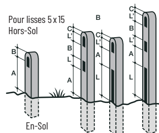
Clôture avec 2 lisses et dalle 0,25 m ou 0,50 m Section 12 x 12 Hauteur hors-sol 1,25 m ou 1,50 m
